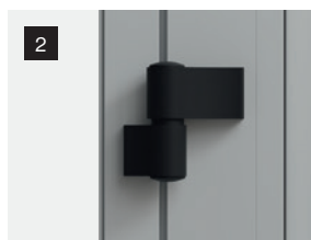
Paumelle aluminium réglable (noir, blanc ou de couleur)
