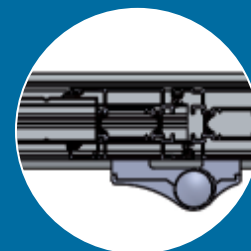
Dormant rupture de pont thermique
