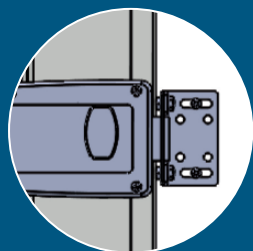
Serrure 1 point bouton poussoir, porte PVC 24
