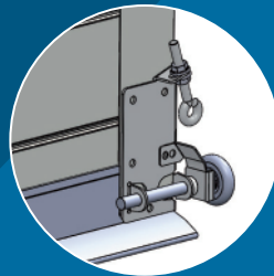
Système d'équilibrage
