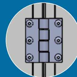
Charnière acier laquée, porte PVC 28 et Alu 27
