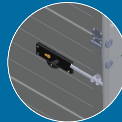
Tringle en acier galvanisé diamètre 15 mm
