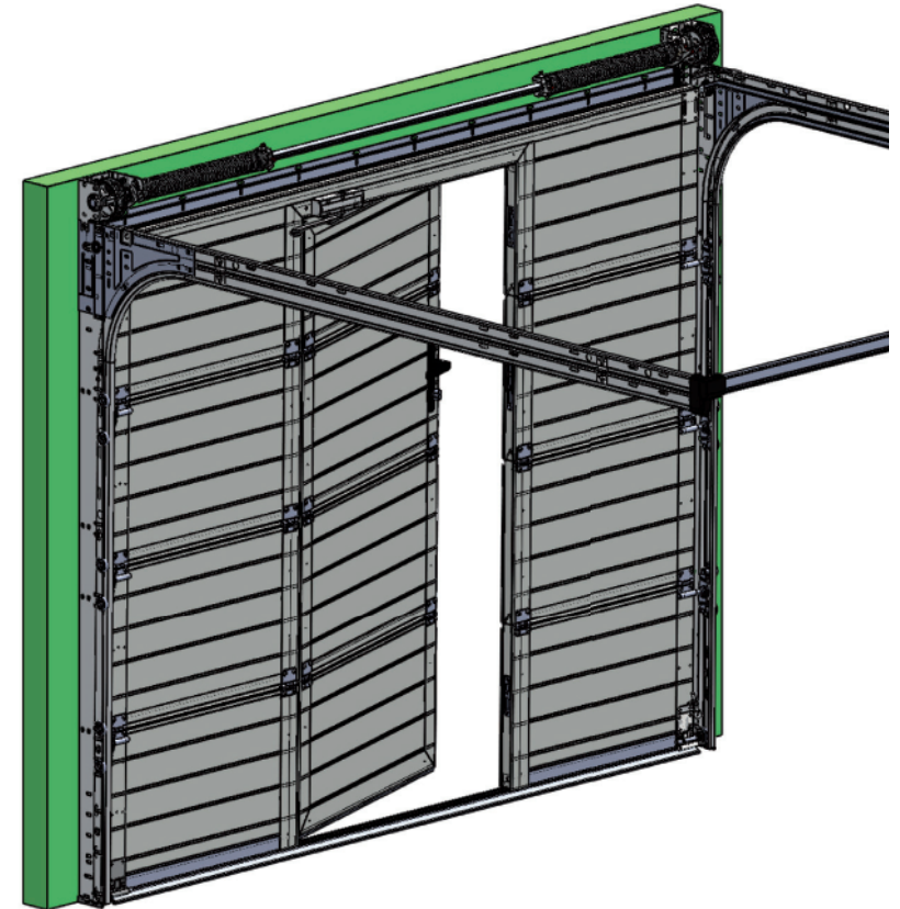
Etanchéité maximale : un joint périphérique et un joint d'amortissement (anti-claquement)
