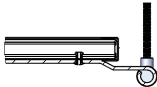
Penture rivetée (sans contre penture) pour porte Alu
