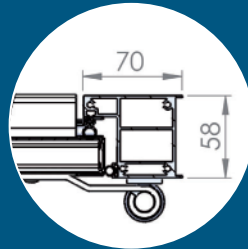
Dormant Alu
