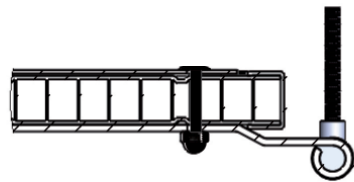
Penture contre penture pour porte PVC
